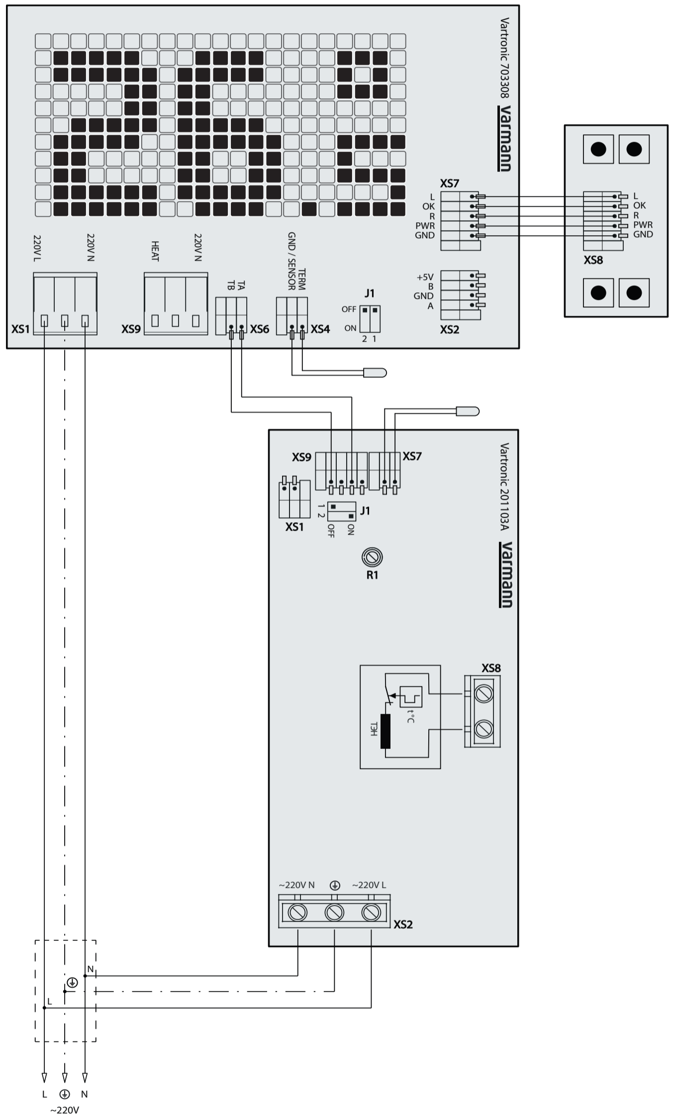
Схема подключения конвекторов Solido Electro и Solido Glass Electro с ручной схемой регулирования.
